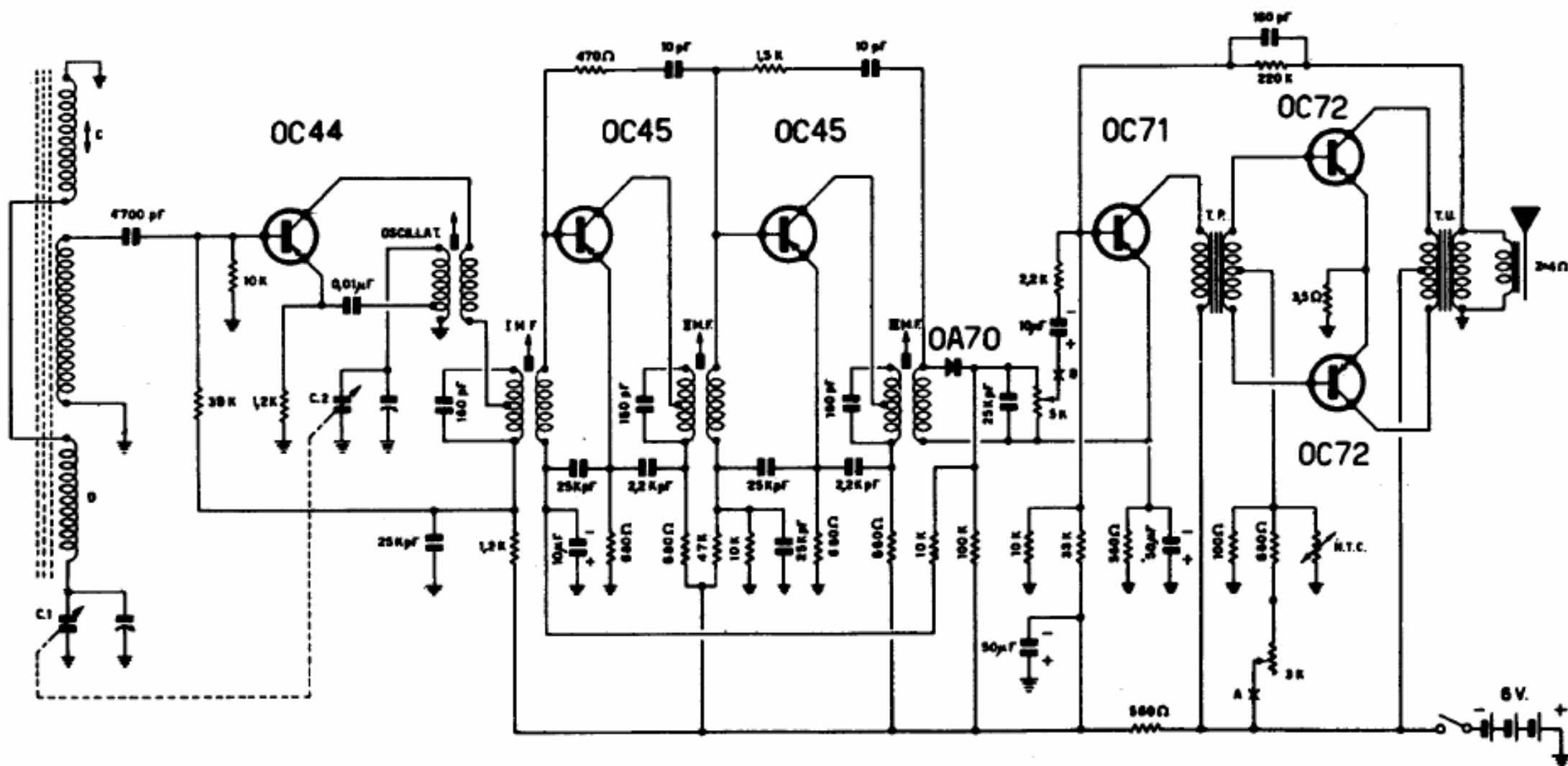
CASTELFRANCHI G.B. - Modello SM 3350. Apparecchio portatile a transistor fornito in scatola di montaggio. Il pannello è a circuiti stampati. Gamma onde medie. Funziona con antenna magnetica incorporata. È provvisto di stadio finale in centrofase, con resa d'uscita di 400 milliwatt. Media frequenza a 468 kc/s. Funziona con due pile da 6 volt, in parallelo. Consuma 8 mA a riposo.
